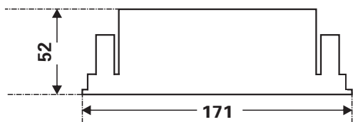
图1:横截面图尺寸
