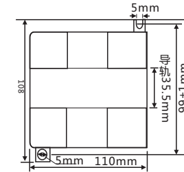
图2：TC-4A4V/4V4V-T类底部装配图
