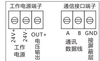
图3：电源、通讯接线
