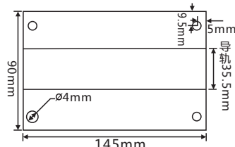
图4：TC-8V4V (-K) 类底部装配图
