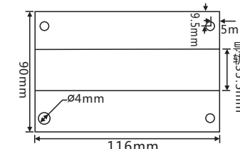
图5：TC-4V4V类底部装配图
