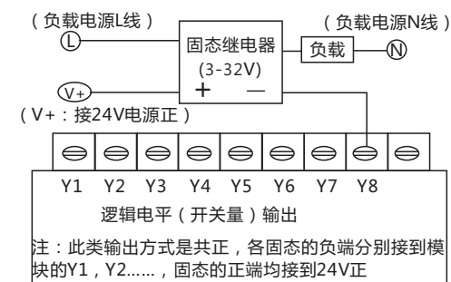
图8:逻辑电平输出型控制固态继电器的输出端口接线说明（也适用于辅助输出端口接线）
