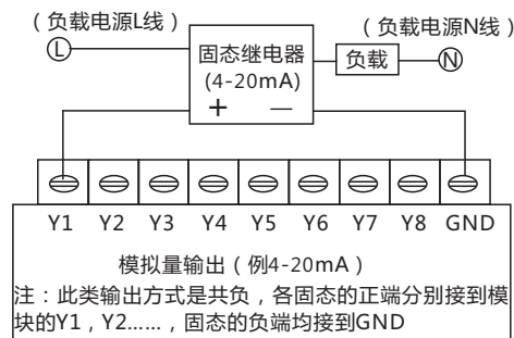
图7:模拟量输出型输出端口接线说明
