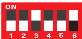
图6地址9时的拨码开关图中“白色”代表开关柄所在位置
