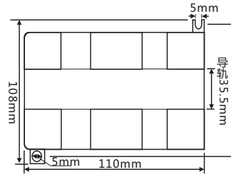
图1：TC-8A8V/8V8V (-T) 类底部装配图
