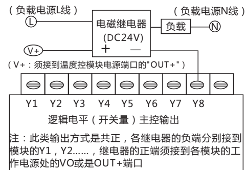
图9:逻辑电平输出型控制电磁继电器的输出端口接线说明（也适用于辅助输出端口接线）
