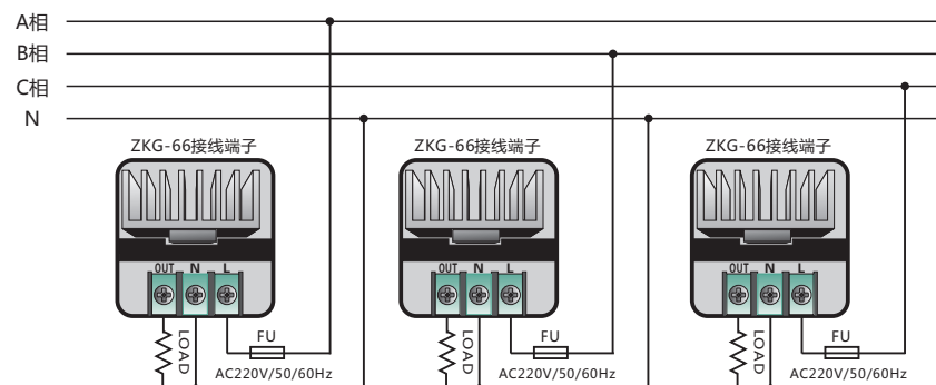
三相接线图:
