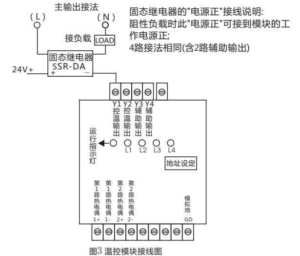
图3 温控模块接线图
