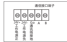
图2 工作电源输入和通讯端口接线
